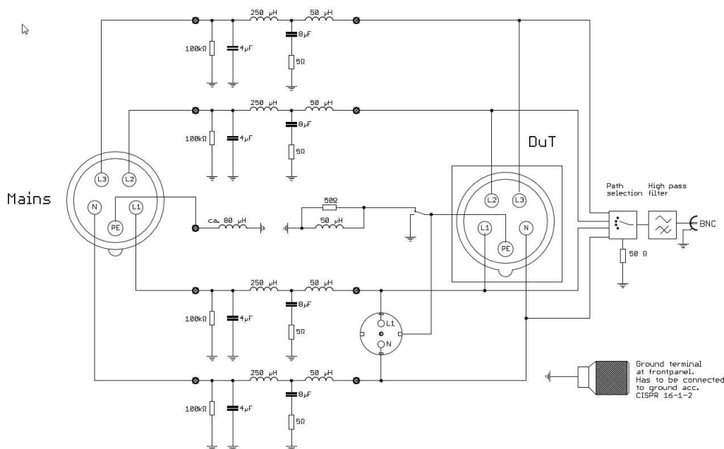
Abb. 2 Funktionsschaltbild Functional diagram
