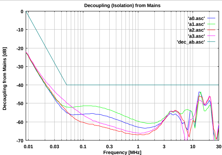
Abb. 9 Entkopplung vom Speisenetz (CEKON-Prüflingsklemmen), BNC mit 50 \Omega Abschluss Decoupling from supply net (CEKON), BNC terminated with 50 \Omega
