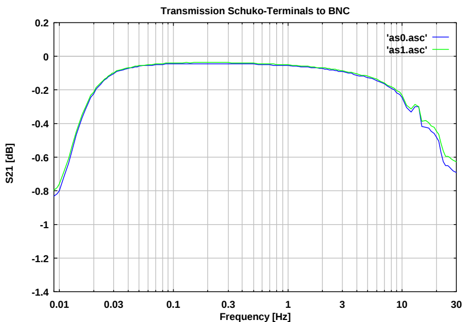
Abb. 6 Transmission Prüflingsklemmen Schuko – BNC Transmission Schuko - BNC
