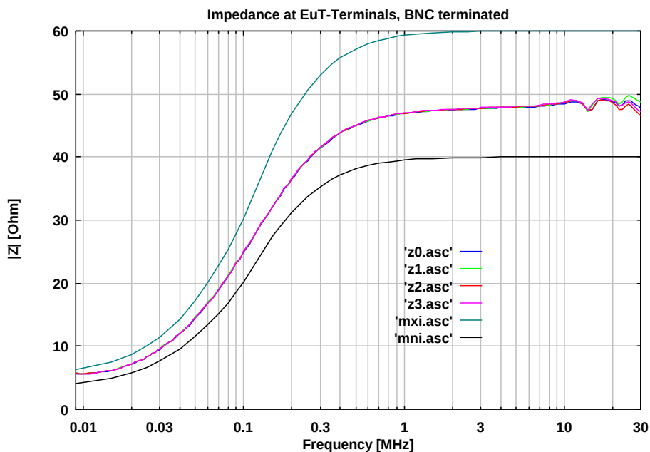
Abb. 4 Impedanz an den Prüflingsklemmen (CEKON), BNC mit 50 \Omega Abschluss Impedance of connector for DuT (CEKON), BNC terminated with 50 \Omega
