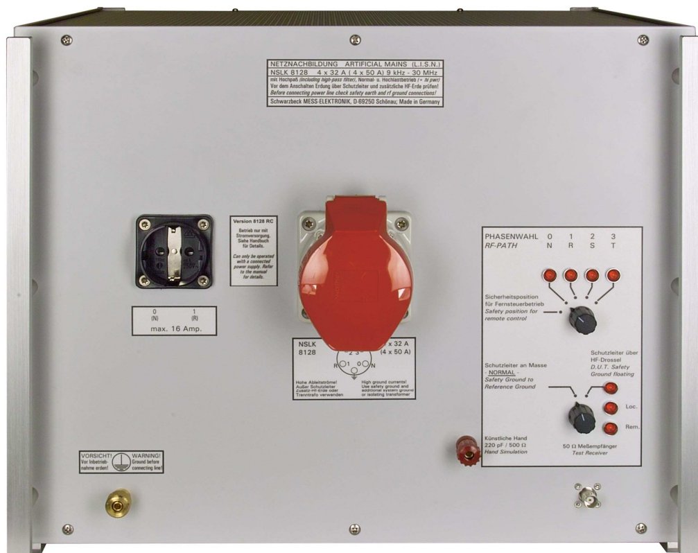
Abb. 1 NSLK 8128 mit Option RC NSLK 8128 with option RC
