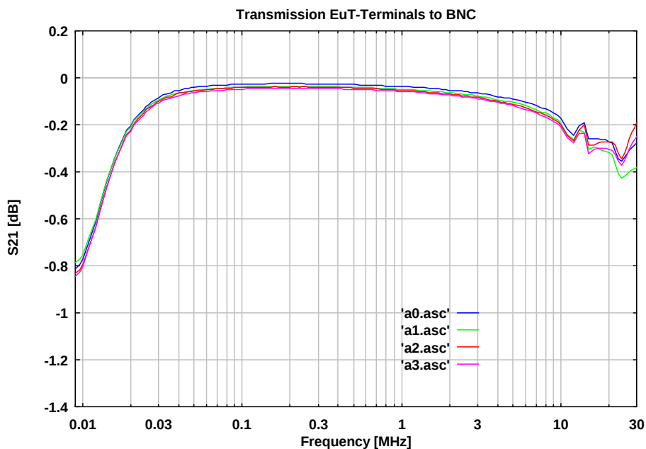
Abb. 3 Transmission Prüflingsklemmen (CEKON) - BNC Transmission CEKON - BNC
