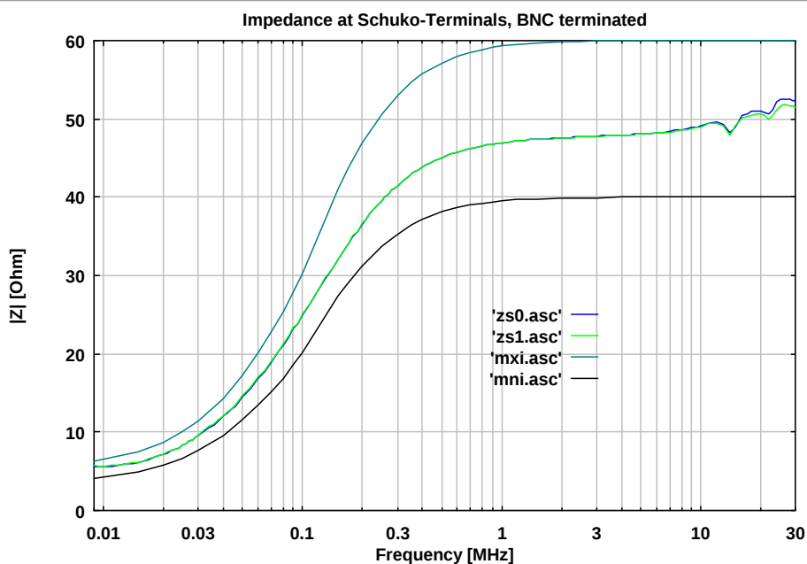
Abb. 7 Impedanz an den Prüflingsklemmen (SCHUKO), BNC mit 50 \Omega Abschluss Impedance of connector for DuT (Schuko), BNC terminated with 50 \Omega
