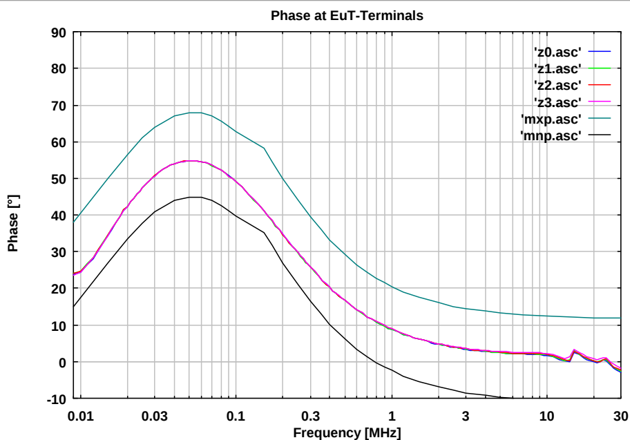
Abb. 5 Phase an den Prüflingsklemmen (CEKON), BNC mit 50 \Omega Abschluss Phase at the connector for DuT (CEKON), BNC terminated with 50 \Omega
