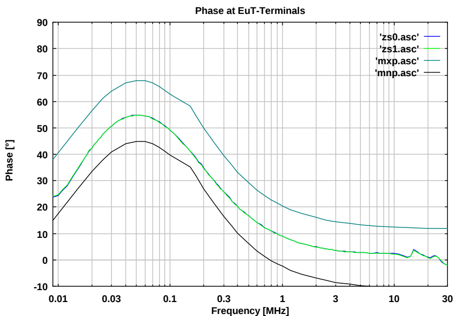
Abb. 8 Phase an den Prüflingsklemmen (SCHUKO), BNC mit 50 \Omega Abschluss Phase at the connector for DuT (Schuko), BNC terminated with 50 \Omega
