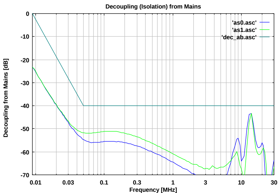
Abb. 10 Entkopplung vom Speisenetz (SCHUKO-Prüflingsklemmen), BNC mit 50 \Omega Abschluss/ Decoupling from supply net (Schuko), BNC terminated with 50 \Omega
